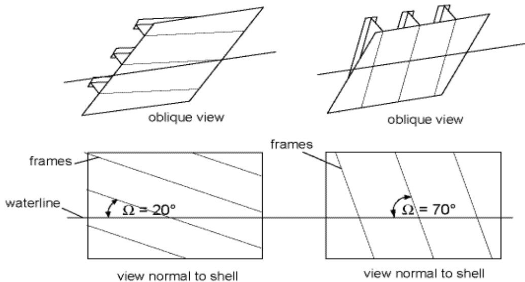
Figure 6 : Shell Framing Angle Ω (1/3/2008)
